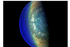
木星内部喷射气流
